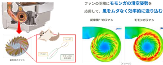
ネイチャーテクノロジー「モモンガファン」の乾燥の風量アップの説明
