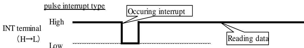
Fig.11 Interrupt output (pulse interrupt type)
