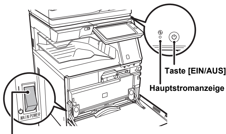
Hauptschalter
